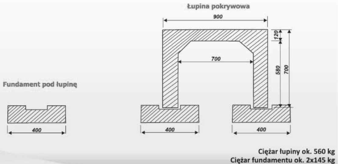
Rys. Pokrywy do zabezpieczenia kanalizacji kablowej
